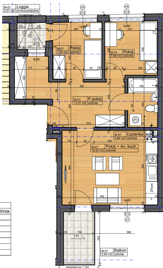
Rzut lokalu w skali 1:100
