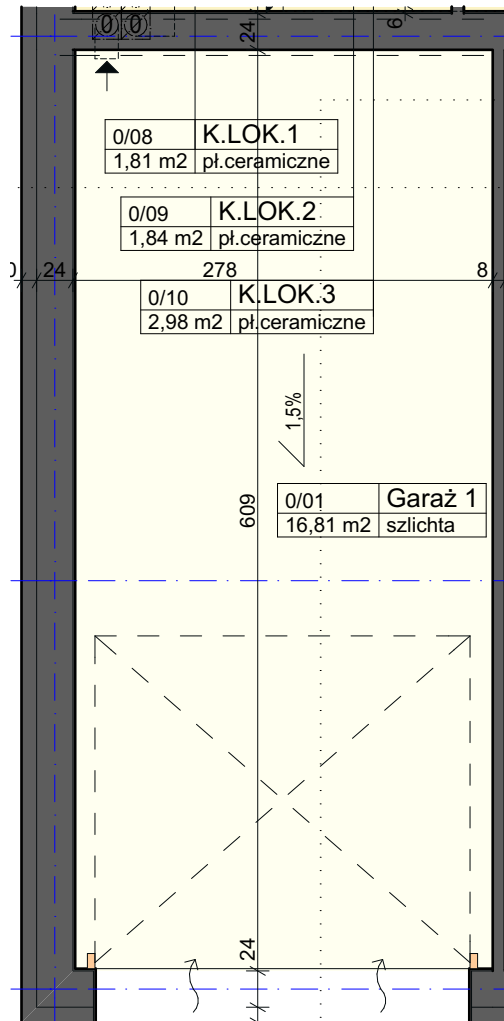
Rzut lokalu w skali 1:50
