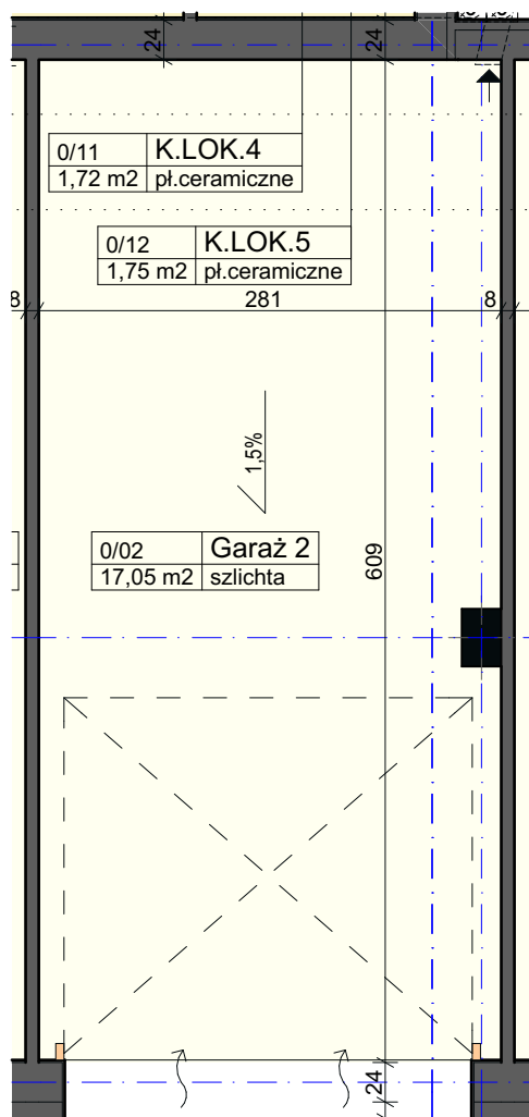
Rzut lokalu w skali 1:50
