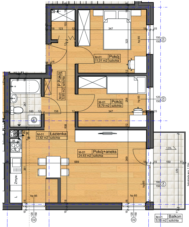
Rzut lokalu w skali 1:100
