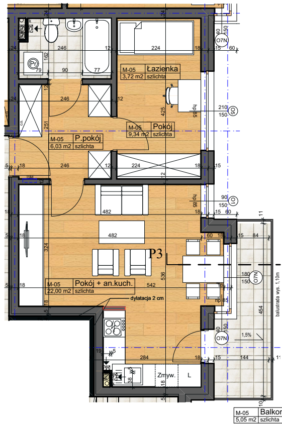
Rzut lokalu w skali 1:100
