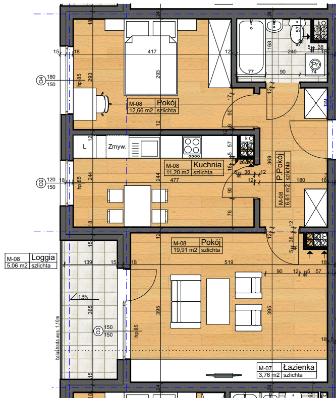
Rzut lokalu w skali 1:100
