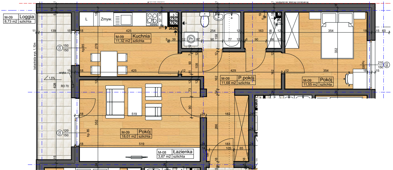
Rzut lokalu w skali 1:100
