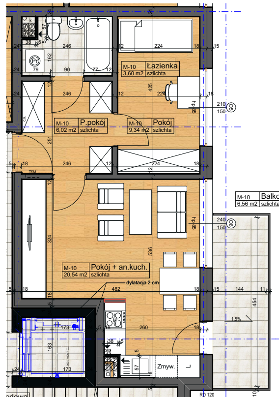
Rzut lokalu w skali 1:100
