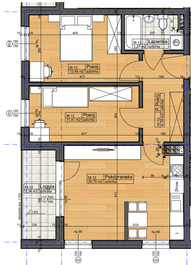
Rzut lokalu w skali 1:100
