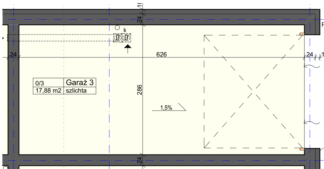
Rzut lokalu w skali 1:50
