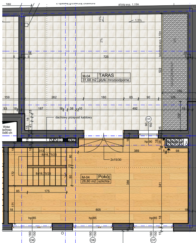
Rzut drugiego poziomu w skali 1:100
