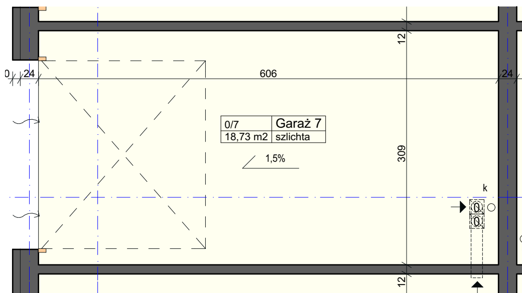
Rzut lokalu w skali 1:50
