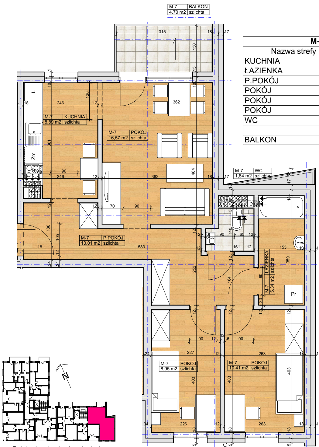
Rzut lokalu w skali 1:75
