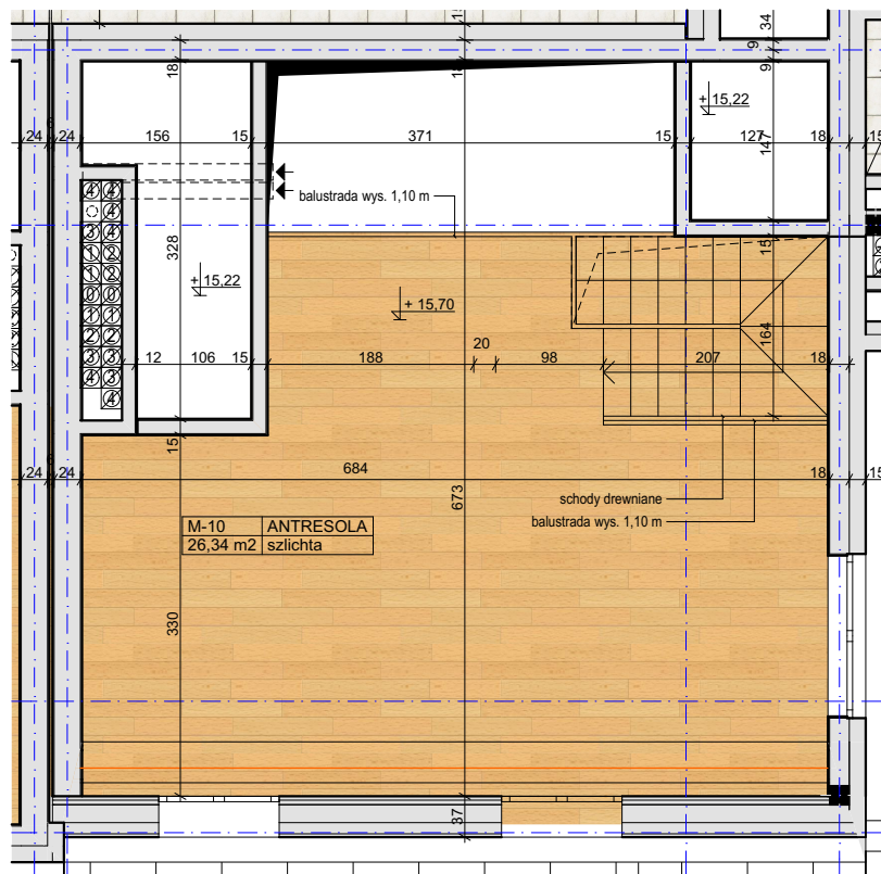
Rzut lokalu w skali 1:75
