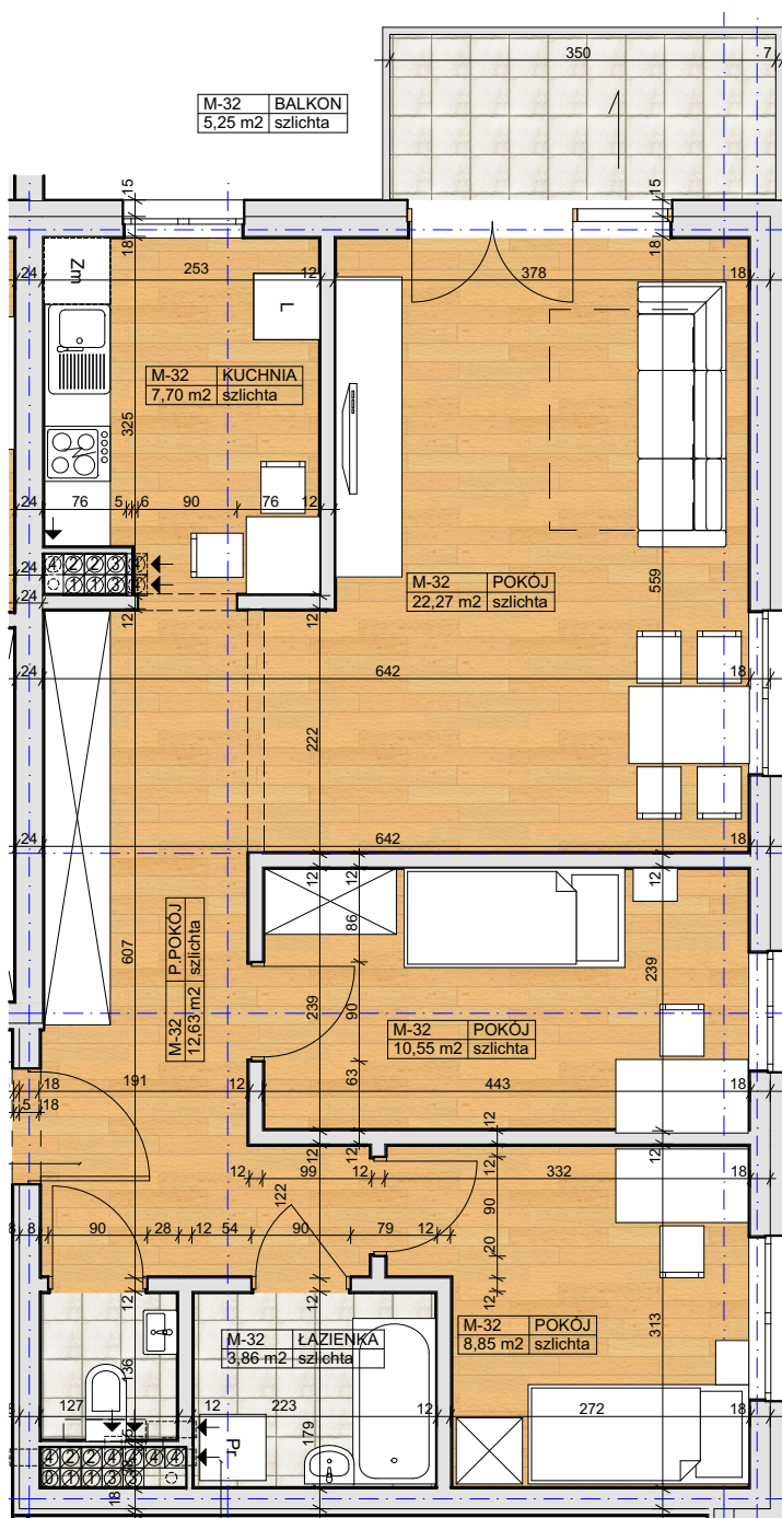
Rzut lokalu w skali 1:75
