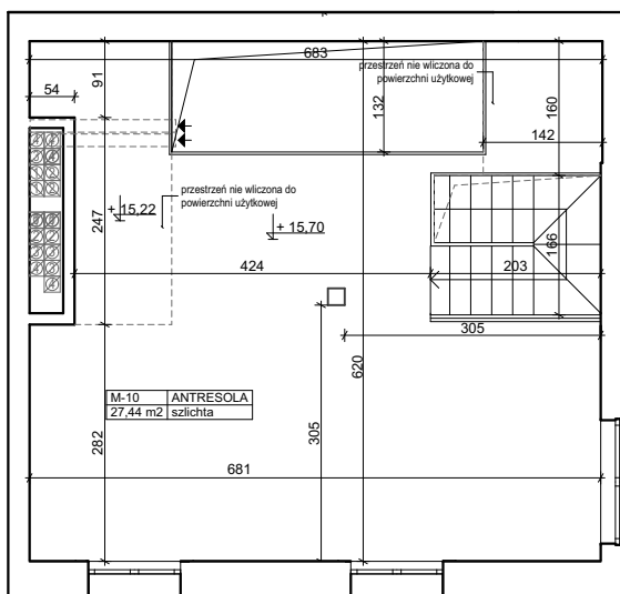
Rzut antresoli 1:100
